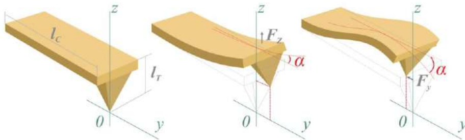
Рисунок 2 – Распределение нормальных и латеральных сил, воздействующих на АСМ-кантилевер при его изгибе.
