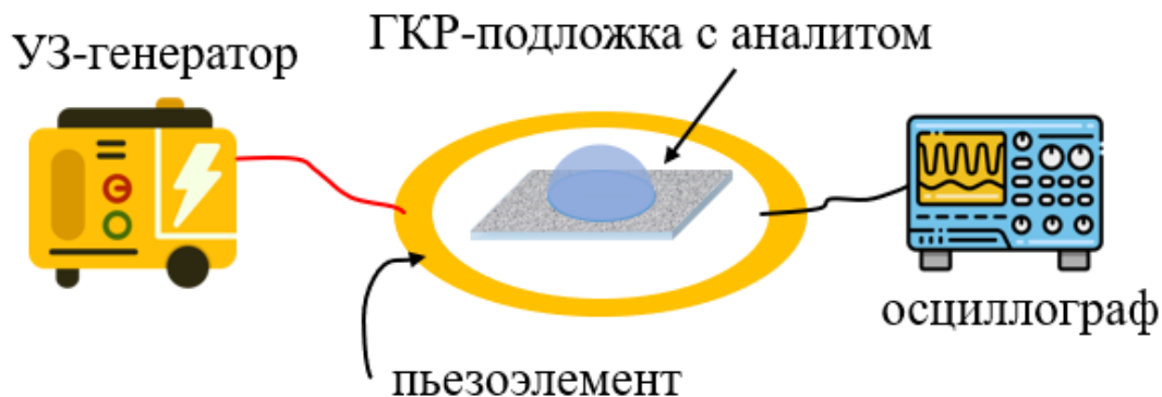
Рисунок 2.8 – Схема эксперимента по проведению пробоподготовки образцов миоглобина с помощью ультразвука
