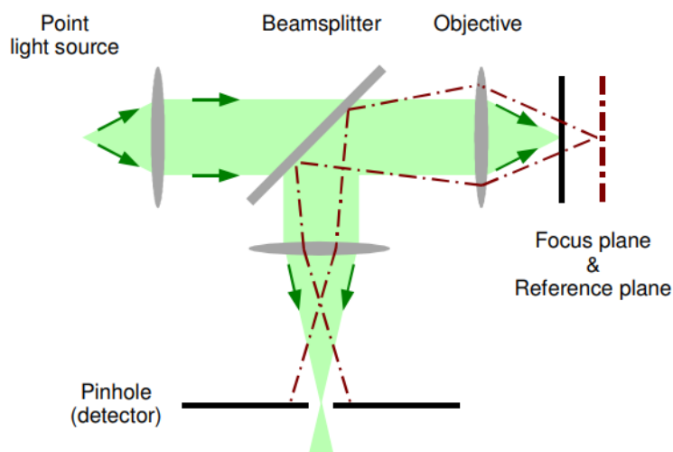
Рисунок 2.4 – Принципиальная схема оптического пути конфокального микроскопа
