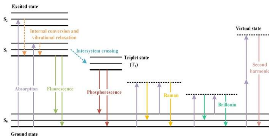
Рисунок 1.1 – Диаграмма Яблонского [4]
