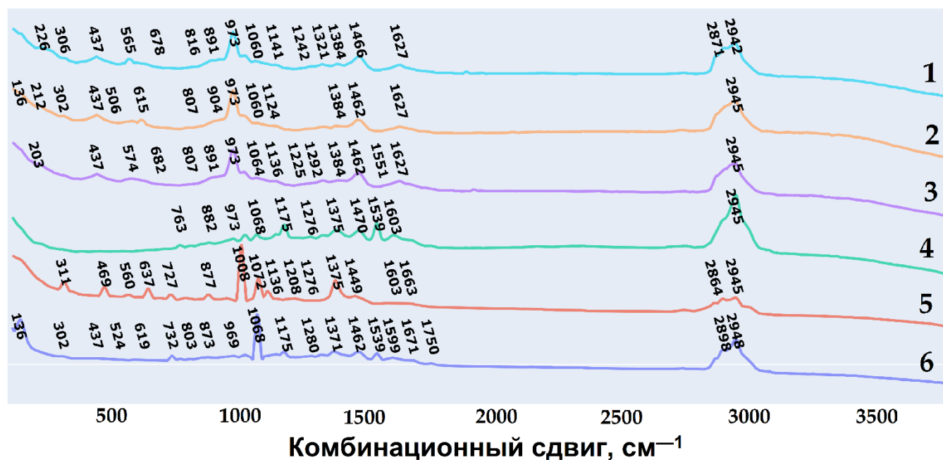
Рисунок 5.1 – Усредненные спектры олигосахаридов после предварительной обработки: (1) oligo-a-(1-2)-Man, (2) oligo-b-(1-3)-Glc, (3) oligo-b-(1-6)-Glc, (4) oligo-DHG-Ef, (5) oligo-GI-Kp, (6) oligo-GM-Af
