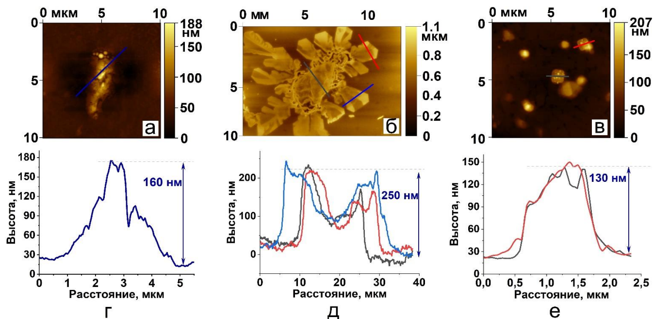
Рисунок 4.3 – Типичные изображения аморфных агломератов: (а) АСМ изображение Типа 1; (б) оптическое изображение кристалла Типа 2; (в) АСМ изображение кристаллических точек Типа 3 и соответствующие профили сечений (г, д, е). На АСМ и оптическом изображениях линиями указаны прямые, вдоль которых извлекался профиль сечения. Цвет линии соответствует цвету профиля
