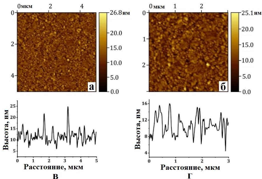
Рисунок 2.1 – АСМ изображения ГКР-подложек Ag#G: (а) 5x5 мкм, (б) 3x3 мкм; (в, г) соответствующие профили сечения
