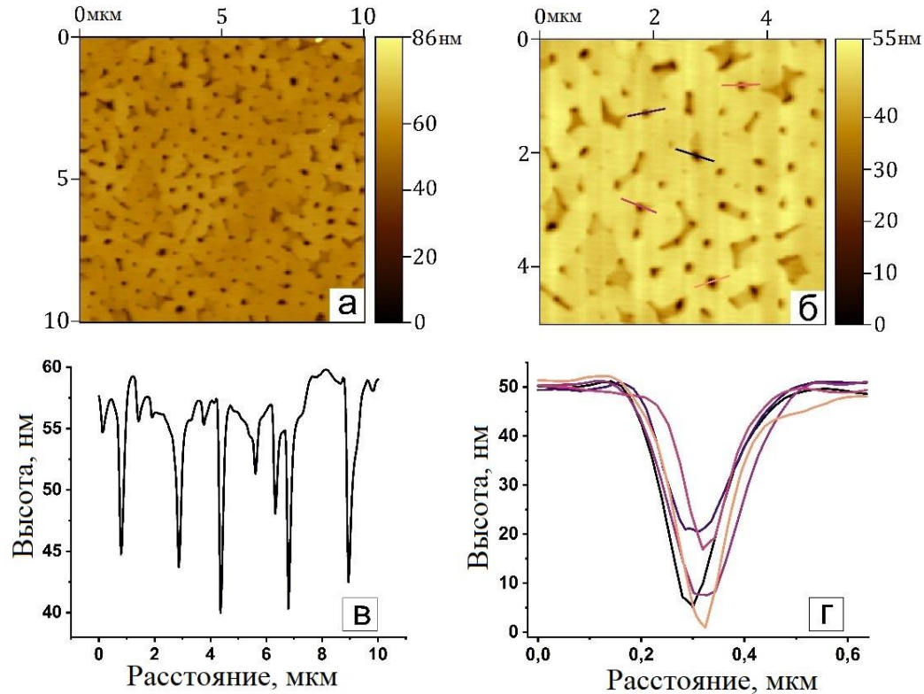
Рисунок 2.2 – АСМ изображения ГКР-подложек Ag#M: (а) 10x10 мкм; (б) 5x5 мкм; (в, г) соответствующие профили сечения
