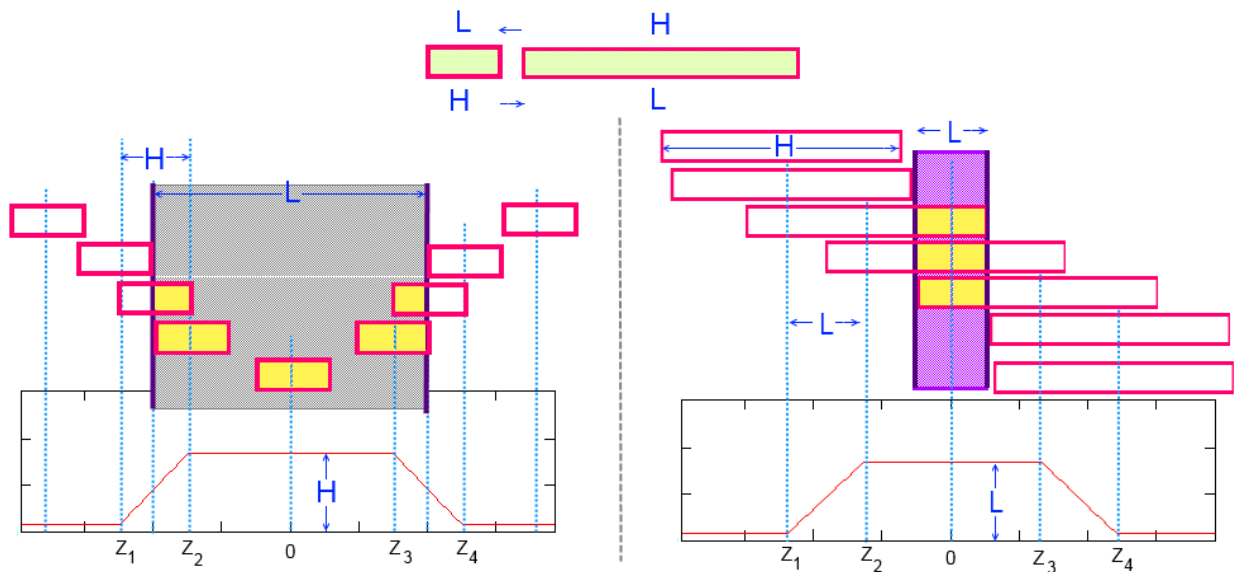
Рисунок 3.1 – Свёртки прямоугольных профилей аппаратной функции (ширина H ) и образца (ширина L ) для двух случаев: (i) H < L (слева) и (ii) H > L (справа)
