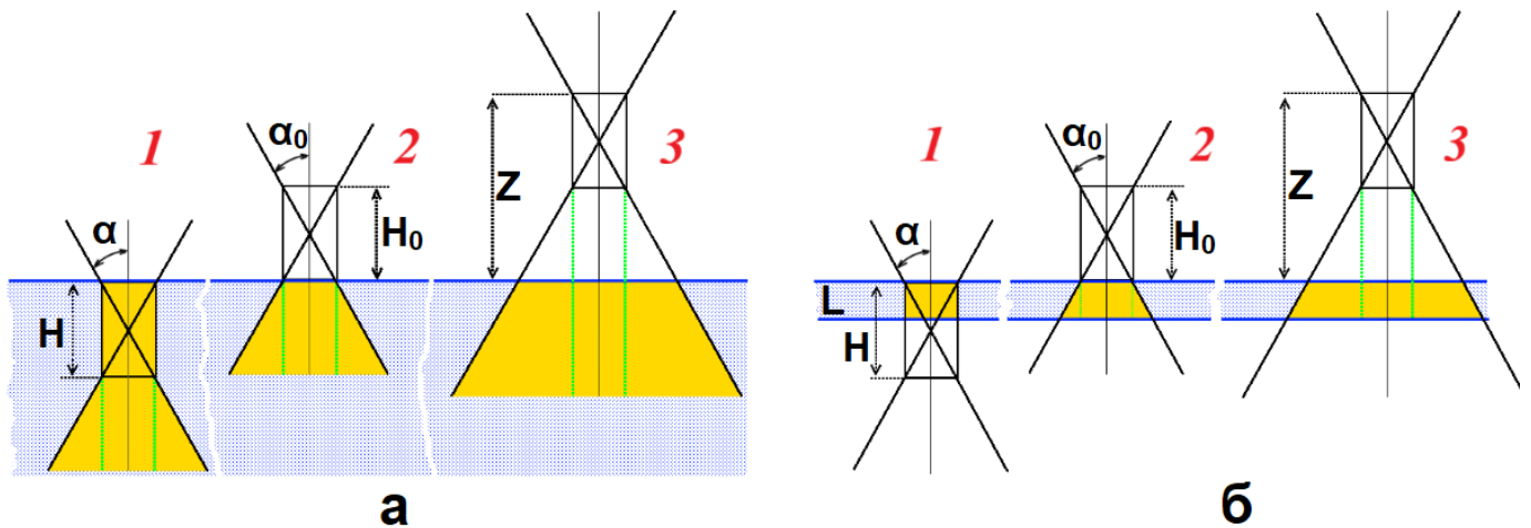
Рисунок 3.3 – Положения измерительного цилиндра относительно образца для модели (а) толстого и (б) тонкого слоя
