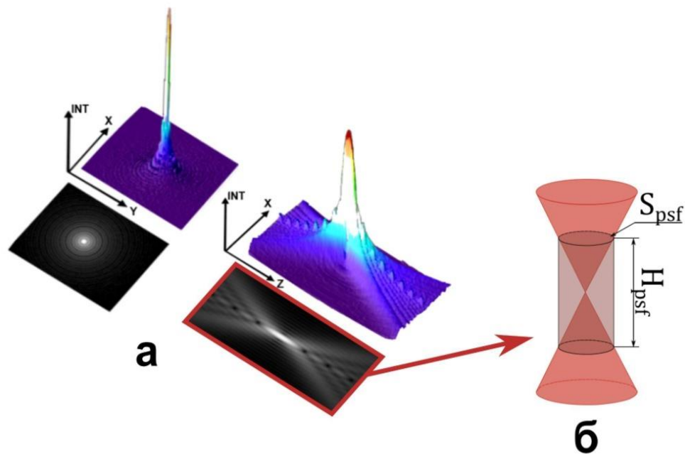
Рисунок 2.5 – (а) PSF конфокального микроскопа в латеральном и аксиальном направлениях; (б) схематичное представление измерительного цилиндра конфокального микроскопа
