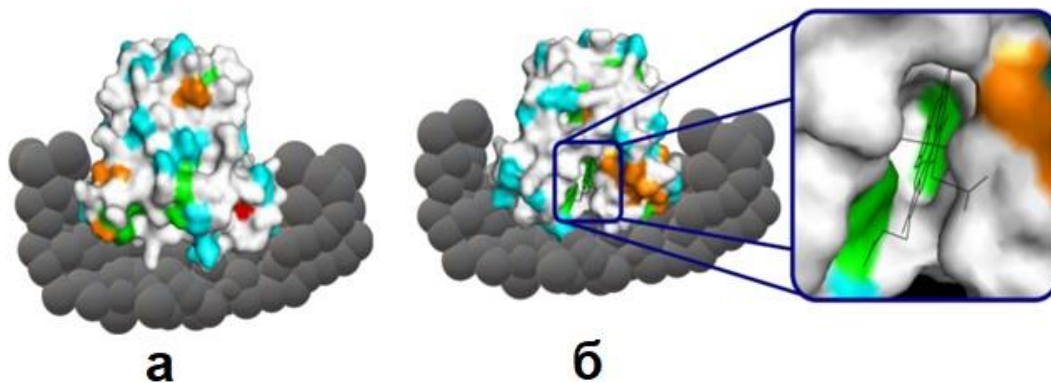
Рисунок 4.2 – Предполагаемая ориентация молекул миоглобина относительно Ag ГКР-активного субстрата при воздушной сушке: (а) вид спереди и (б) вид сзади. Красный — Met; оранжевый — дипептиды Ala–Ala, Leu–Gly, Pro–Leu и Ala–Gln; синий — Asp и Glu; зеленый — Phe, Trp и Tyr. Гем показан в виде скелета
