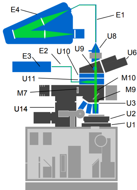
Рисунок 2.3 – Схема спектрометрической системы WiTec Alpha 300R.
