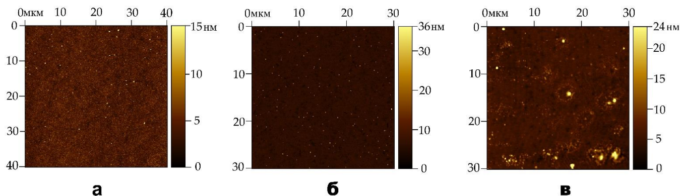
Рисунок 4.4 – АСМ изображения поверхности ГКР-подложек Ag#G (а) без предварительной обработки стеклянной основы и с предварительной обработкой стеклянной основы (б) по методу I, (в) по методу II
