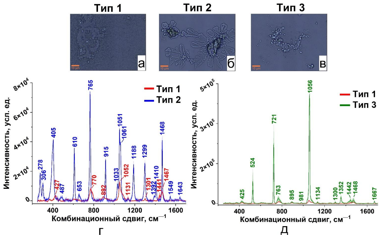
Рисунок 4.1 – Оптическое изображение типов осадков миоглобина: (а) Тип 1 - при высушивании на воздухе; (б) Тип 2 - при высушивании лазером растворов с концентрацией 1 мкг/мл; (в) Тип 3 - при высушивании лазером растворов с концентрацией 10 нг/мл; (г, д) ГКР-спектры, соответствующие каждому типу осадка миоглобина
