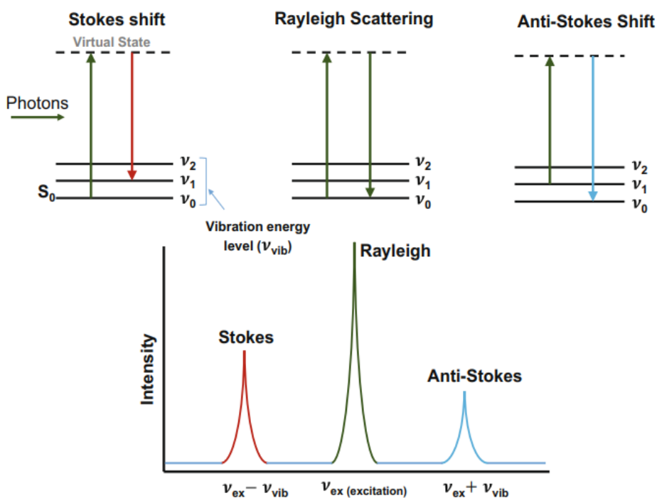
Рисунок 1.2 – Рэлеевское рассеяние в сравнении со Стоксовым и Антистоксовым КР [6]
