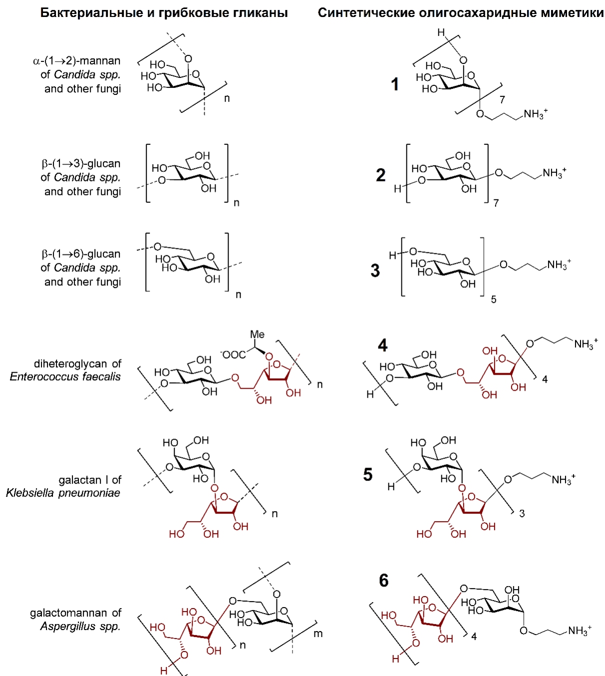
Рисунок 2.7 – Природные бактериальные и грибковые гликаны (слева) и синтетические олигосахаридные миметики (справа)
