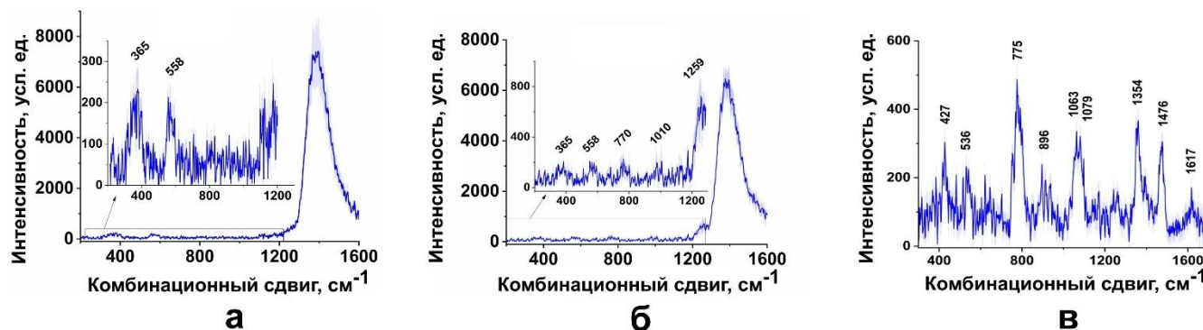
Рисунок 4.6 – (а) КР-спектр покровного стекла, (б) КР-спектр 1 \text{ мг/мл} миоглобина, высушенного на покровном стекле, (в) ГКР-спектр 1 \text{ мкг/мл} миоглобина, высушенного без дополнительного воздействия на подложке Ag#G
