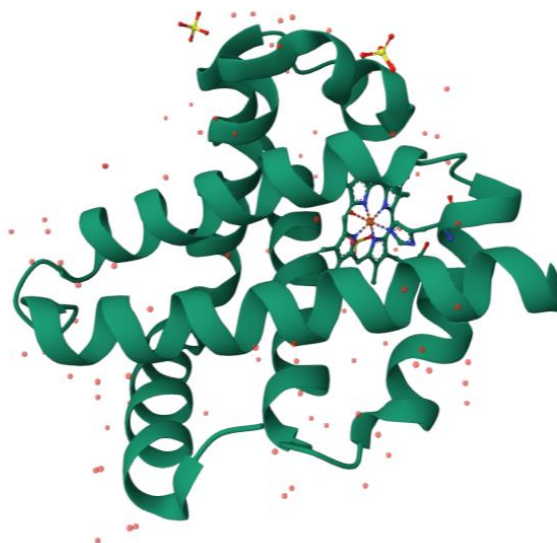
Рисунок 2.6 – Структура молекулы миоглобина. Данные взяты из RCSB Protein Data Bank [193]
