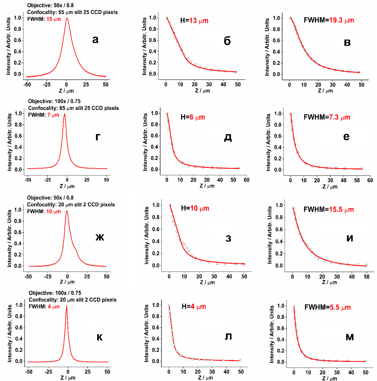
Рисунок 3.4 - Данные RENISHAW [207] (левая колонка: а,г,ж,к), аппроксимация моделью (средняя колонка:б,д,з,л), аппроксимация Лоренцем (правая колонка: в,е,и,м). Длина волны возбуждающего лазера 785 нм, параметры объектива и конфокальность указаны на картинках левой колонки
