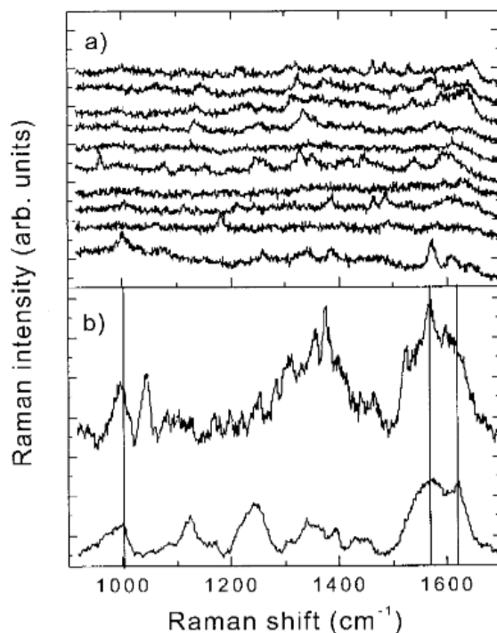
Рисунок 1.4 – (а) ГКР-спектры миоглобина 10^{-11} М в растворе наночастиц серебра, иммобилизованного на поверхности стекла, полученные при времени интегрирования 1 сек. (промежуток между двумя последовательными измерениями 60 сек.); (б) Верхняя кривая - спектр, полученный путем суммирования 100 серий ГКР-спектров, нижняя кривая - спектр комбинационного рассеяния сухого миоглобина (время интегрирования 30 сек.) [106]
