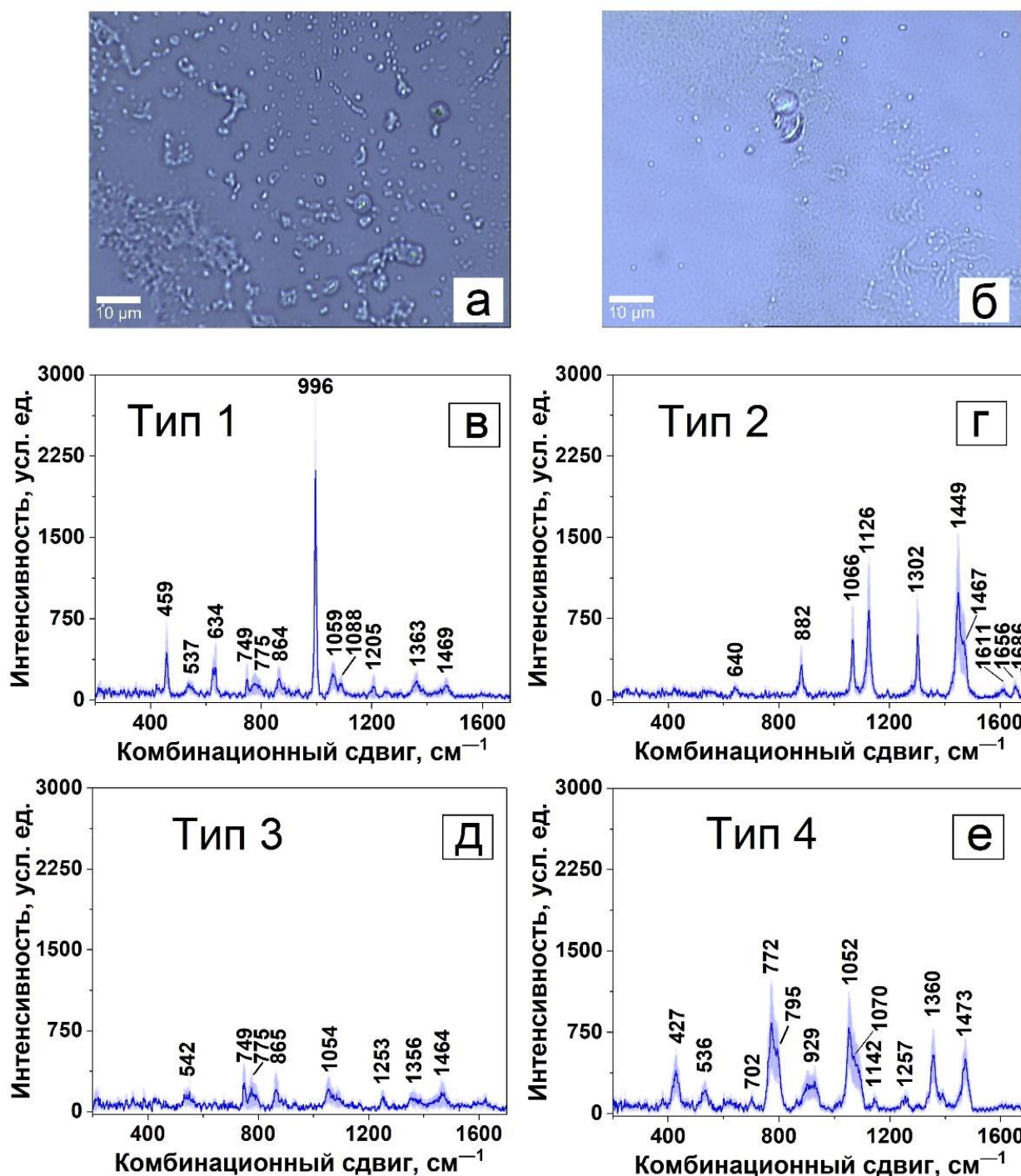
Рисунок 4.5 – Осадок миоглобина после пробоподготовки с использованием ультразвука (47 и 580 кГц). Оптические изображения (а,б); ГКР-спектры: Тип 1 (в), Тип 2 (г), Тип 3 (д), Тип 4 (е)
