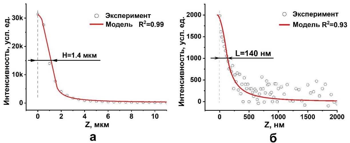
Рисунок 3.6 - Экспериментальные (кружки) и модельные (красные линии) профили Z-скана кремния (а) и азота (б)
