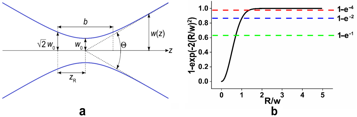
Рисунок 3.2 - (а) Параметры Гауссова пучка; (б) Доля мощности гауссова пучка, содержащаяся в пятне, ограниченном апертурами с различными радиусами
